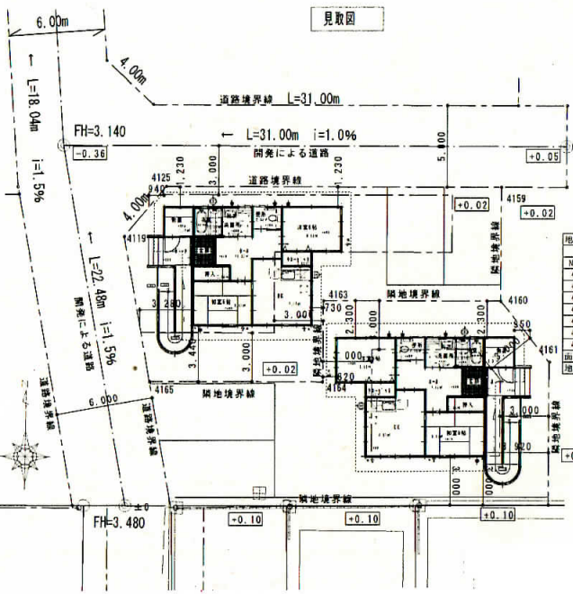
建築場所： 見取図
