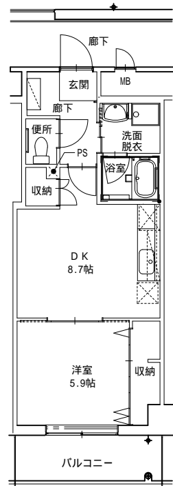
1DK-C (2F)
