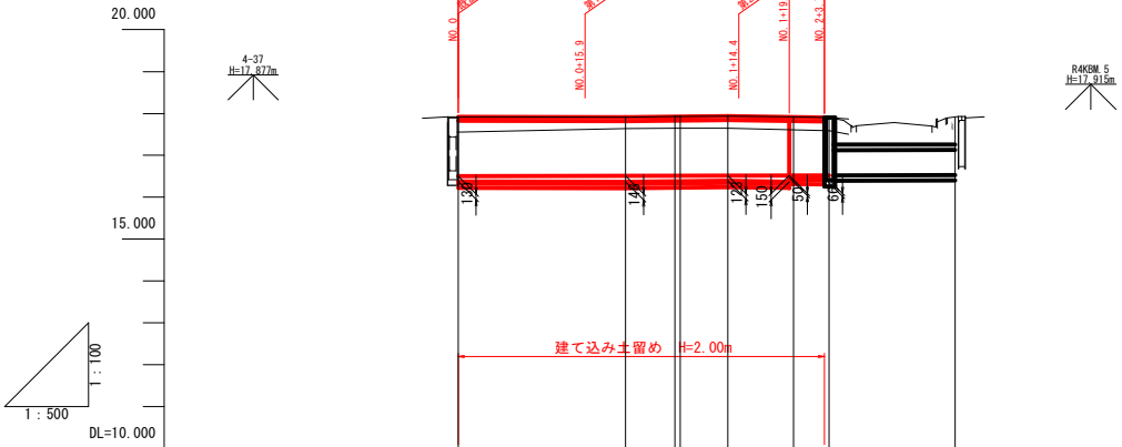
縦断面図
