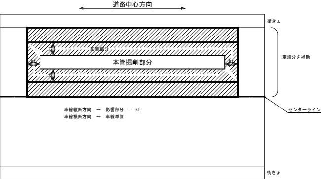
平面図(参考図-1)
