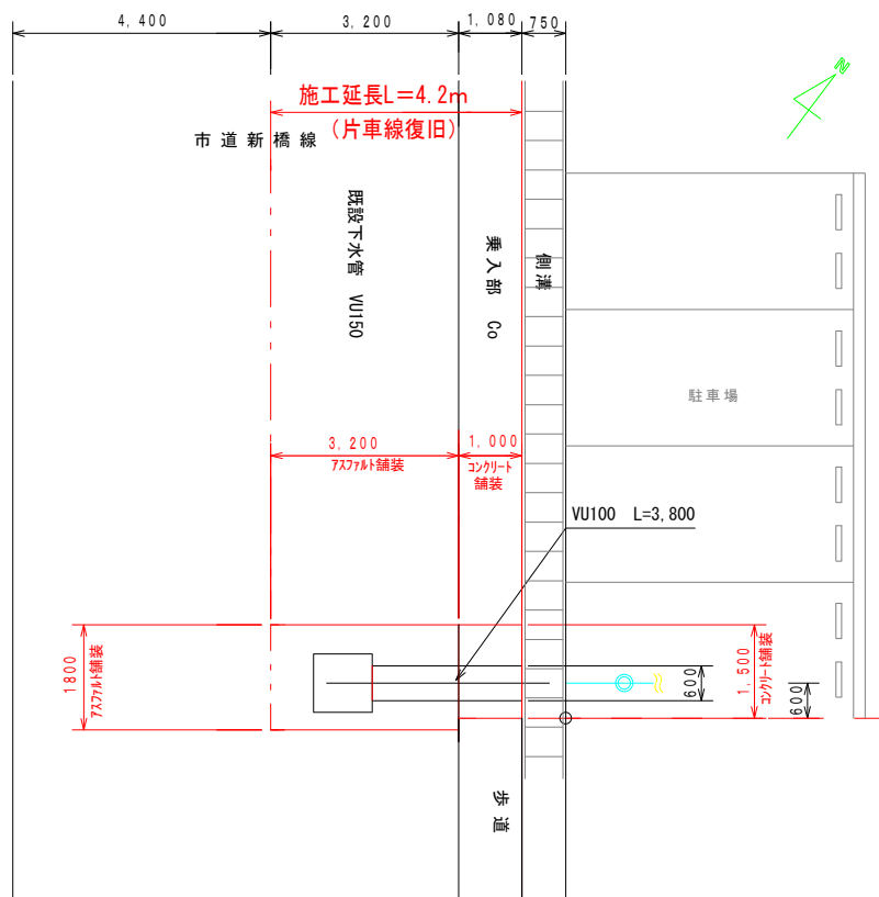
平面図 S=1:100
