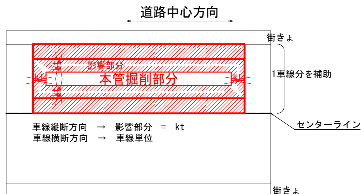
平面図 (参考図-1)
