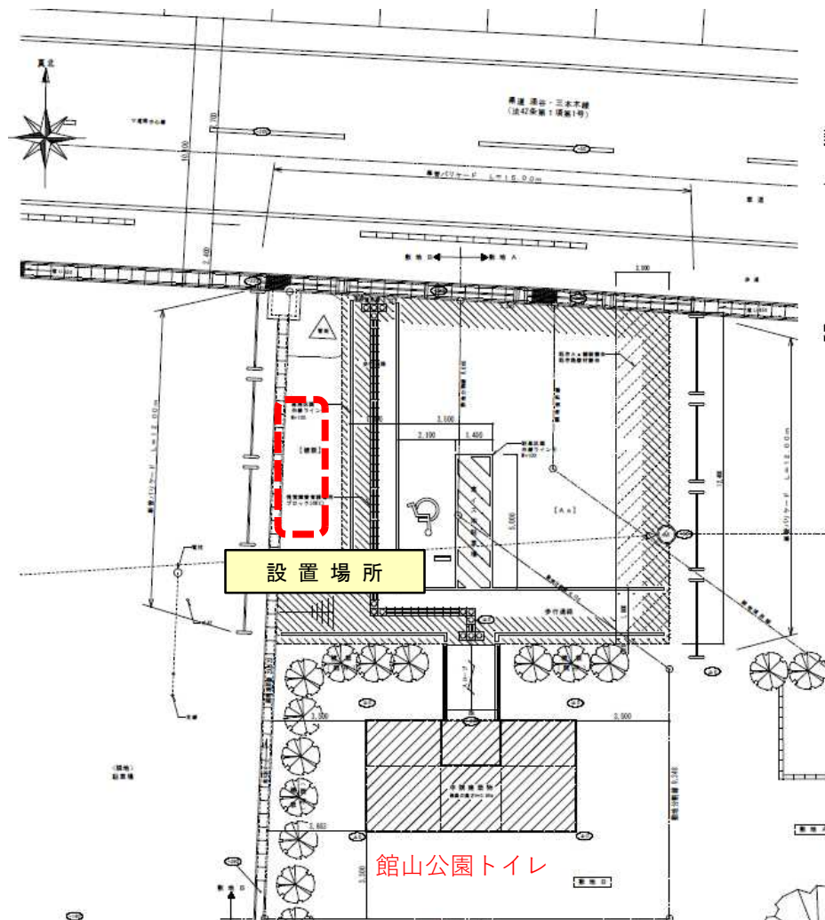
配置図
