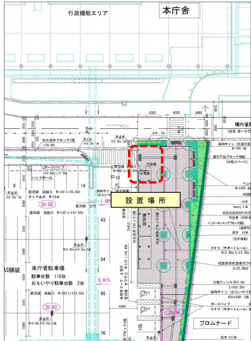
配置図
