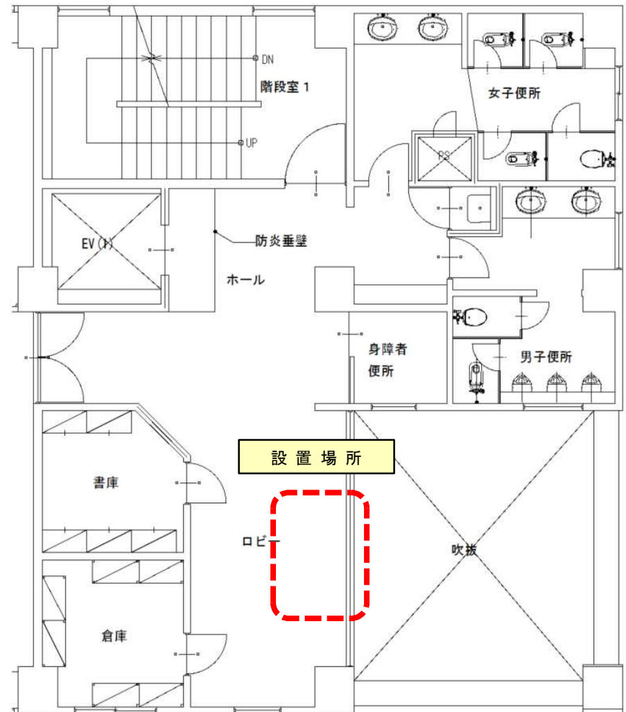
配置図
