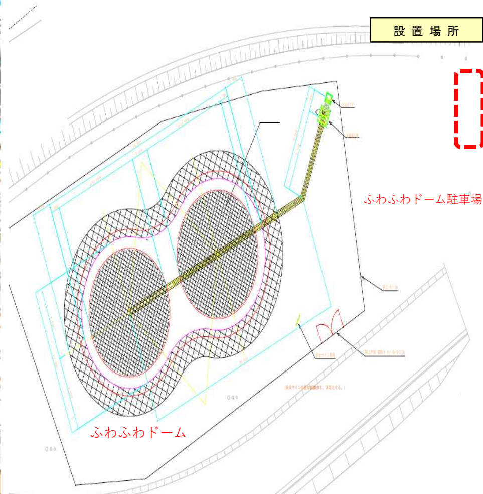
配置図
