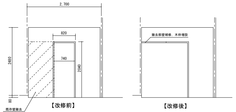
A-A' 展開図
