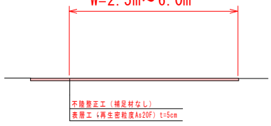
市道朽木橋2号線 標準断面図 W=2.5m~6.0m
