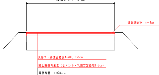
標準断面図
