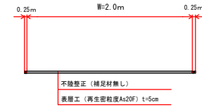
標準断面図
