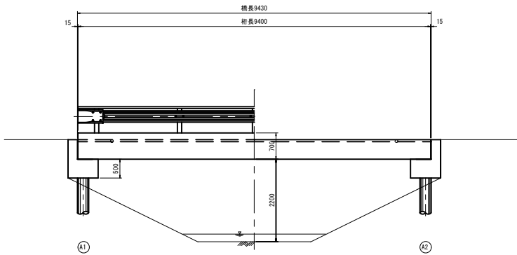
側面図
