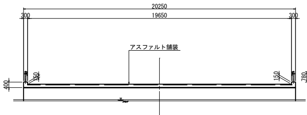
断面図
