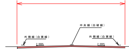
市道小金丁南線2工区 標準断面図
