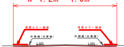
市道小金丁南線1工区 標準断面図
