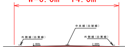
市道南町米倉線 標準断面図
