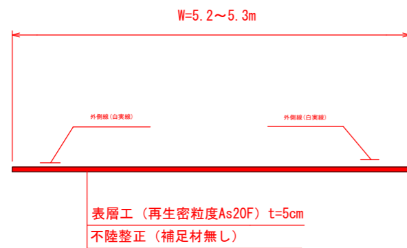
標準断面図
