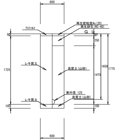
00: 配水管 04: PEφ100 H=1.65 (掘削・埋戻し) 1/25
