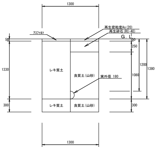
00: 配水管 05: 不断水1 H=1.7 (掘削・埋戻し) 1/25
