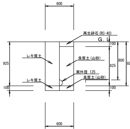
00：配水管 11：PEφ100 H=0.8 (RC10cm) (掘削・埋戻し) 1／2 5
