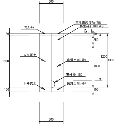
00: 配水管 03: PEφ150 H=1.2 (掘削・埋戻し) 1/2
