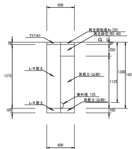
00: 配水管 07: PEφ100 H=1.3 (掘削・埋戻し) 1/2
