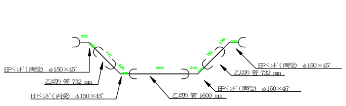
E暗渠詳細図
