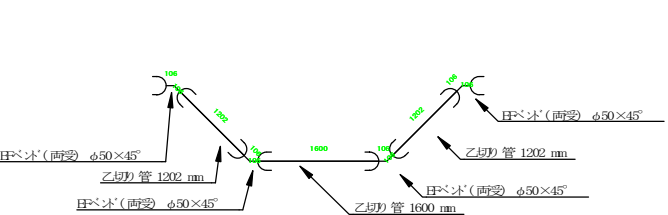
F暗渠詳細図
