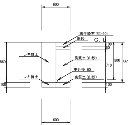
00：配水管 15：排水管 VPφ50 (7ヶ所層) (掘削・埋戻し) 1／2 5
