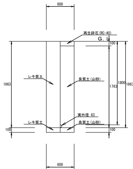
00：配水管 09：PEφ50 H=1.8 (RC10cm) (掘削・埋戻し) 1／2 5
