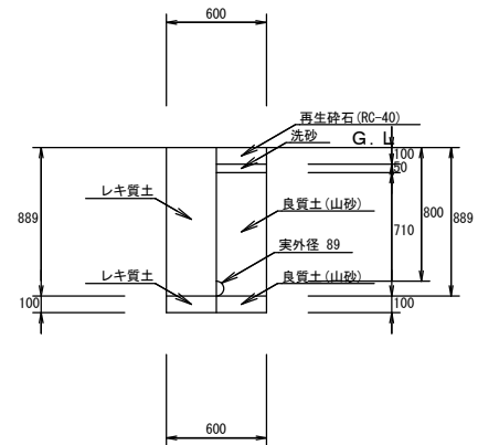
00：配水管 14：排水管 VPφ75 (7ヶ所層) (掘削・埋戻し) 1／2 5
