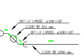
D暗渠詳細図
