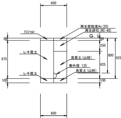
00: 配水管 01: PEφ100 H=0.8 (掘削・埋戻し) 1/25
