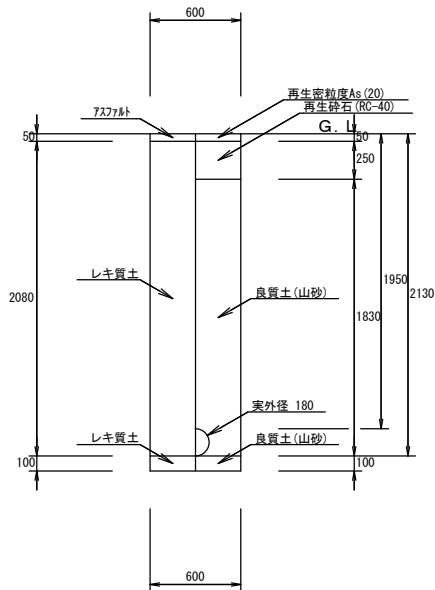
00: 配水管 06: PEφ150 H=1.95 (掘削・埋戻し) 1/2
