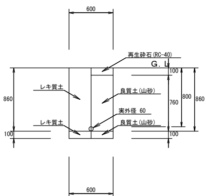
00：配水管 16：排水管 VPφ50 (RC10cm) (掘削・埋戻し) 1／2 5
