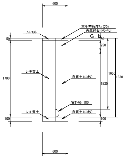
00：配水管 10：PEφ150 H=1.65 (掘削・埋戻し) 1／2 5
