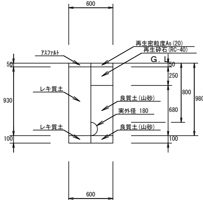
00: 配水管 02: PEφ150 H=0.8 (掘削・埋戻し) 1/25
