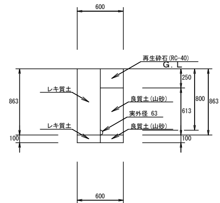
00：配水管 18：乗入 PEφ50 H=0.8 (RC25cm) (掘削・埋戻し) 1／2 5
