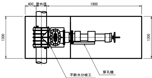
不断水平面図 S=FREE
