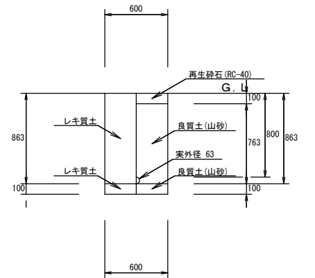
00: 配水管 08: PEφ50 H=0.8 (RC10cm) (掘削・埋戻し) 1/25
