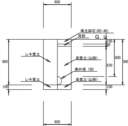
00：配水管 12：PEφ150 H=0.8 (7ヶ所層) (掘削・埋戻し) 1／2 5
