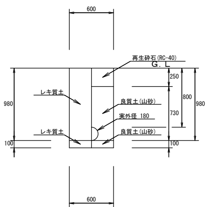
00：配水管 17：乗入 PEφ150 H=0.8 (RC25cm) (掘削・埋戻し) 1／2 5
