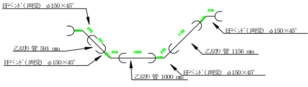
A暗渠詳細図
