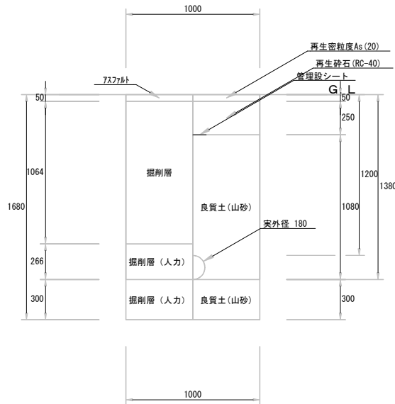
不排水連絡工φ150（掘削・埋戻し） 1／20
