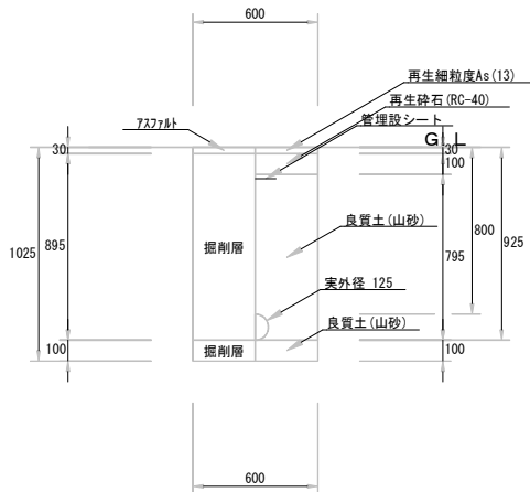
配水管 01: 配水管φ100（歩道部）（掘削・埋戻し） 1／20
