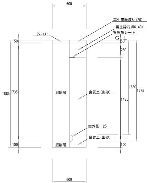
伏越工②（掘削・埋戻し） 1／20
