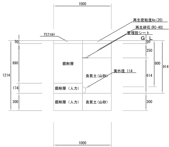
不排水連絡工φ100（掘削・埋戻し） 1／20
