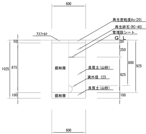
配水管φ100（乗入部）（掘削・埋戻し） 1／20
