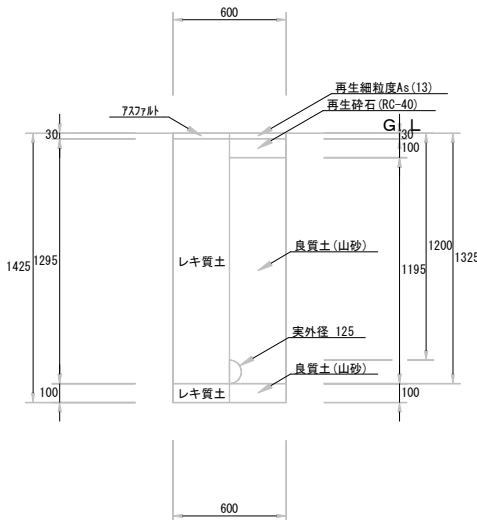
伏越工①（掘削・埋戻し） 1／20
