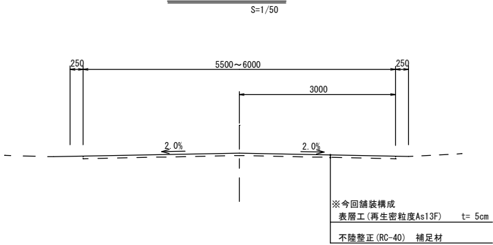
標準断面図
