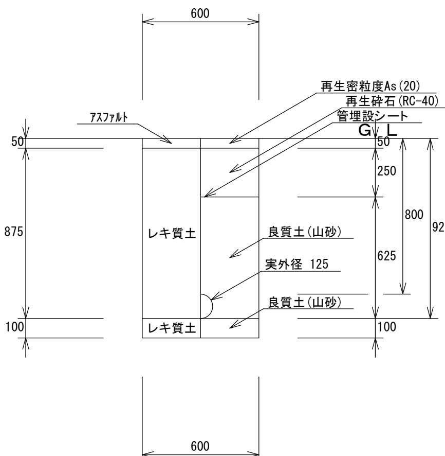
10: PE \phi 100 H=0.8m (As) (掘削・埋戻し) 1/20
