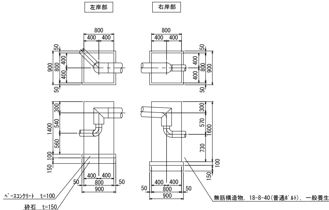
防護コンクリート詳細図 S= 1:60
