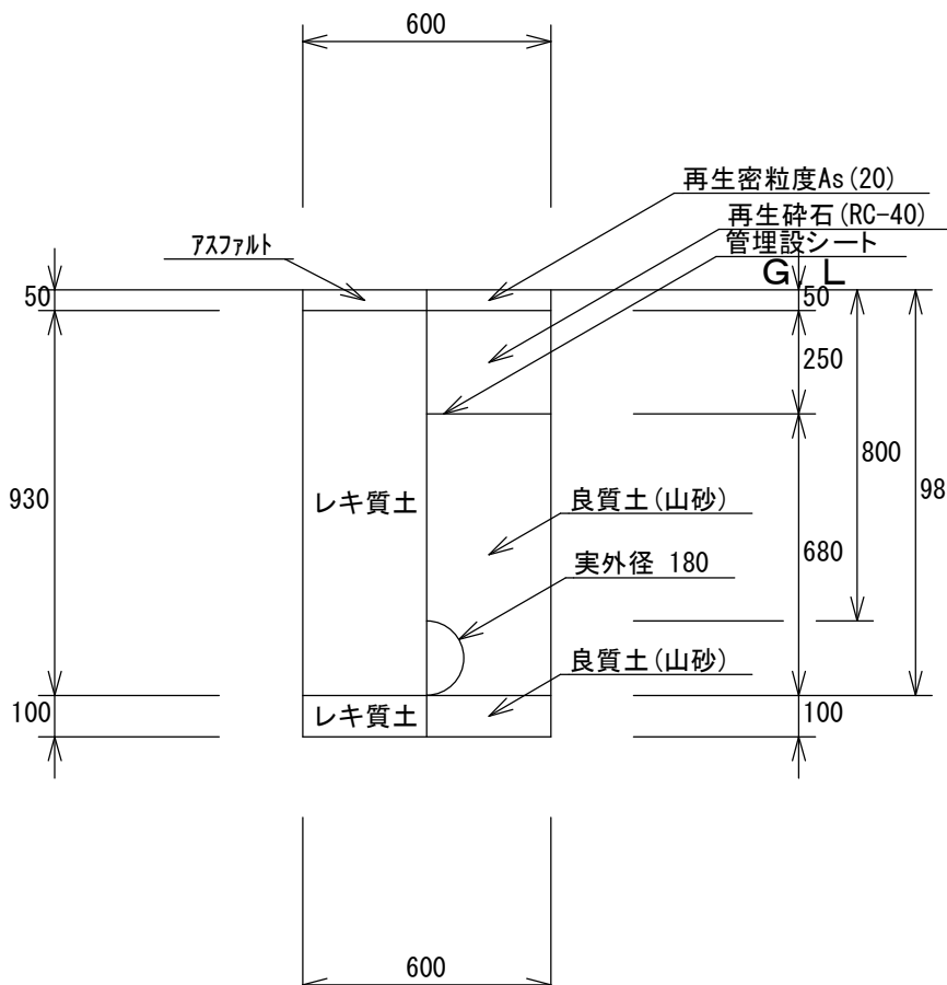
Q1: PE \phi 150 H=0.8m (As) (掘削・埋戻し) 1/20
