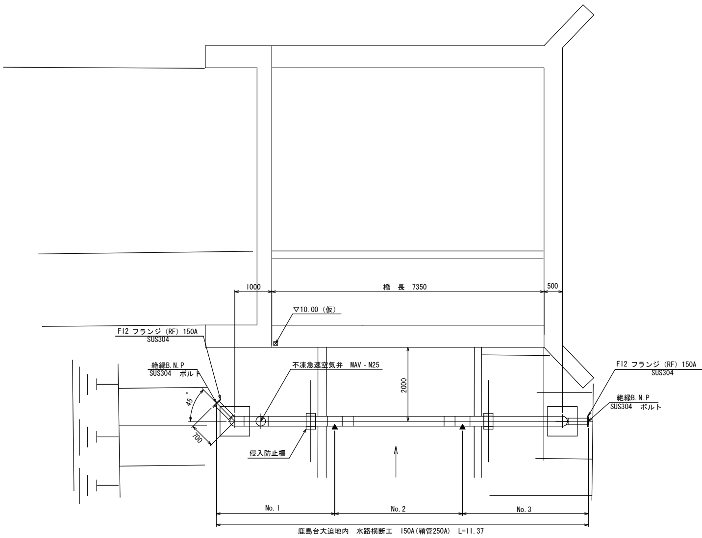
平面図 S= 1:100
