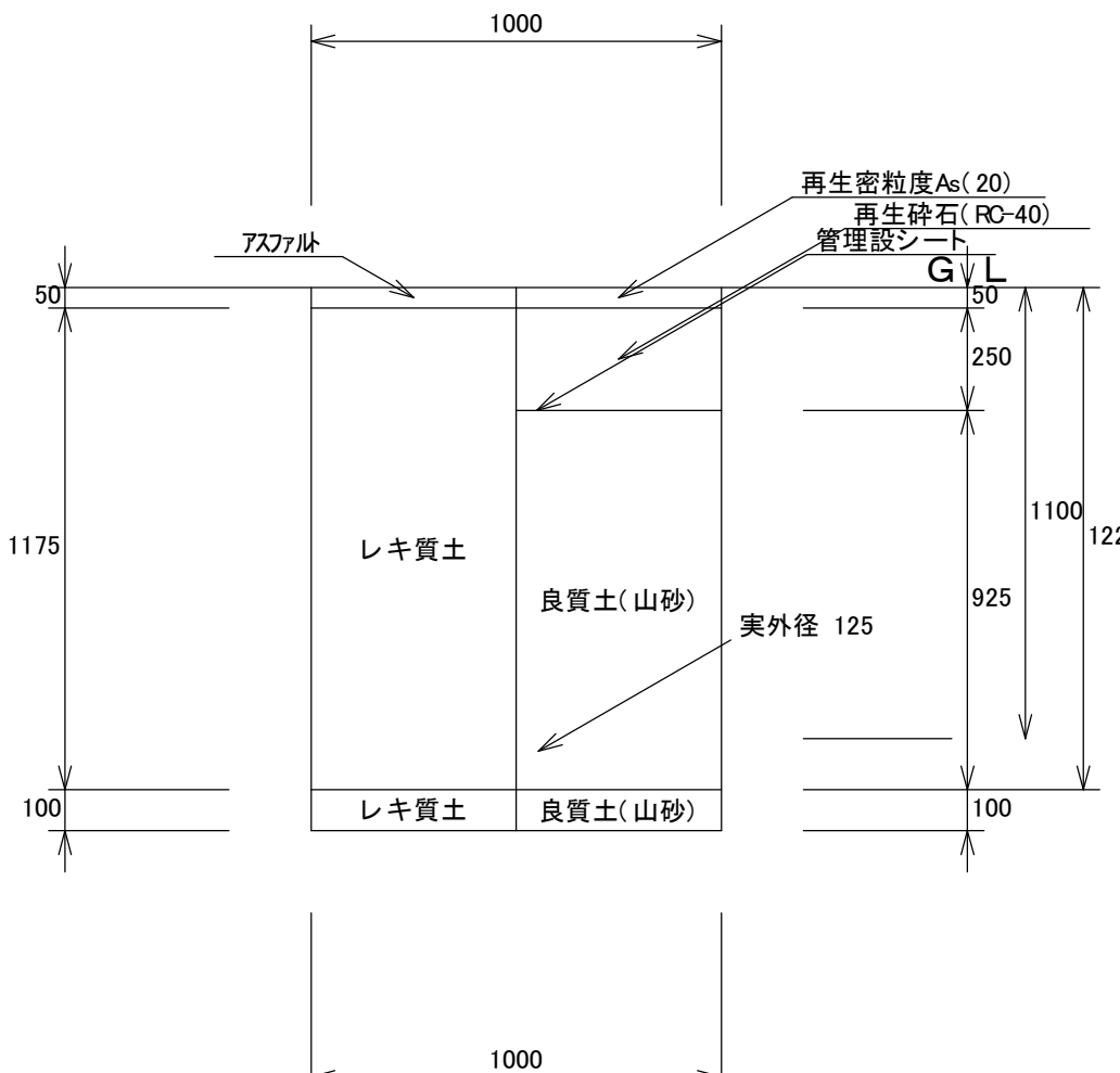
00: 配水管 14: PEφ100 H=1.1m(As) (掘削・埋戻し) 1/2
