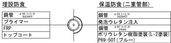
防食詳細図 S=free
