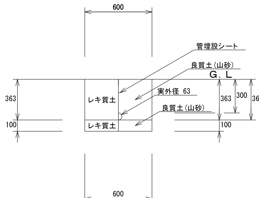
09: VPφ50 H=0.3m (G) (掘削・埋戻し) 1/20
