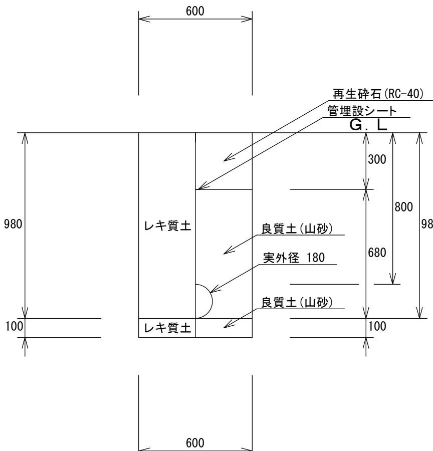
02: PE \phi 150 H=0.8m (C) (掘削・埋戻し) 1/20
