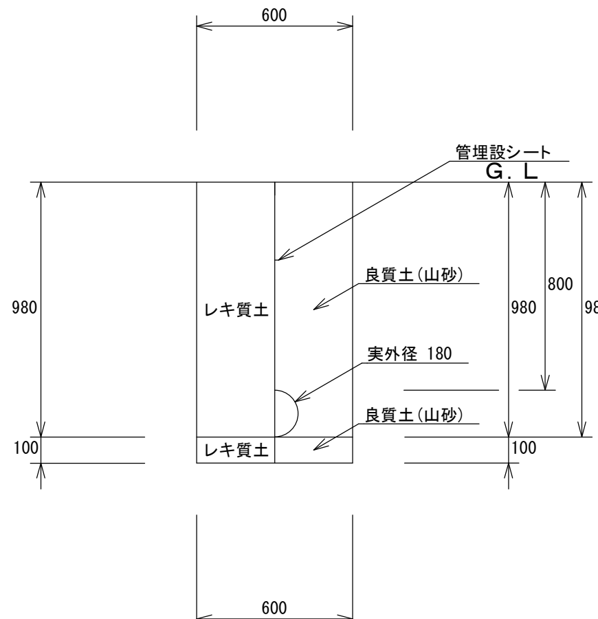
03: PE \phi 150 H=0.8m (G) (掘削・埋戻し) 1/2 C
