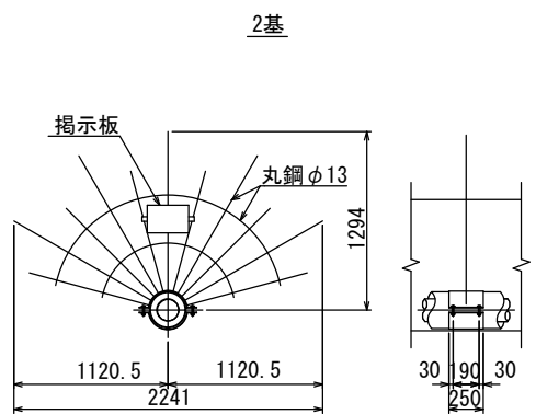
侵入防止柵詳細図 S=1:60
