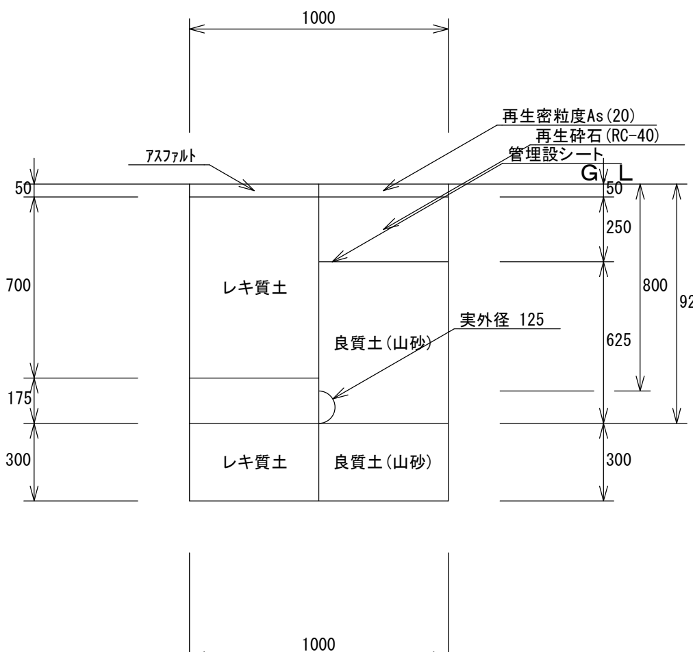
11: 不断水 \phi 125 \times 100 H=0.8m (As) (掘削・埋戻し) 1/20
