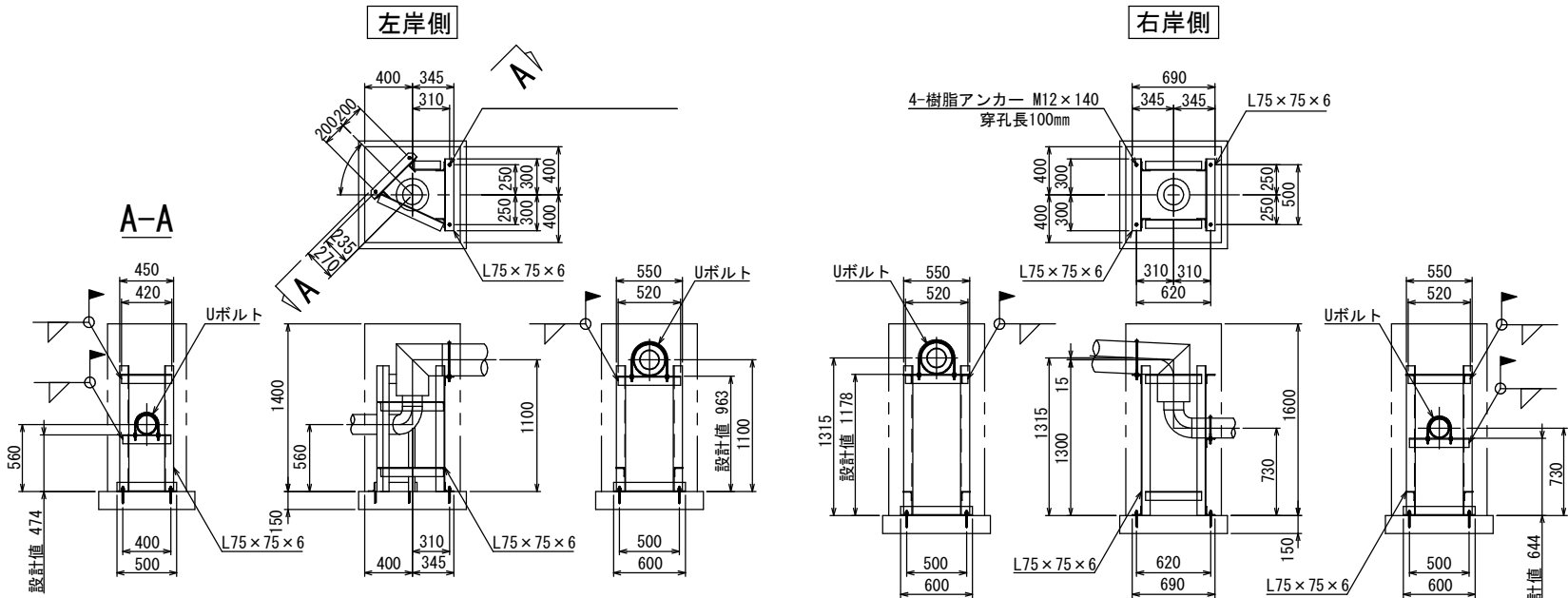
支保工参考図 S=1 : 60
