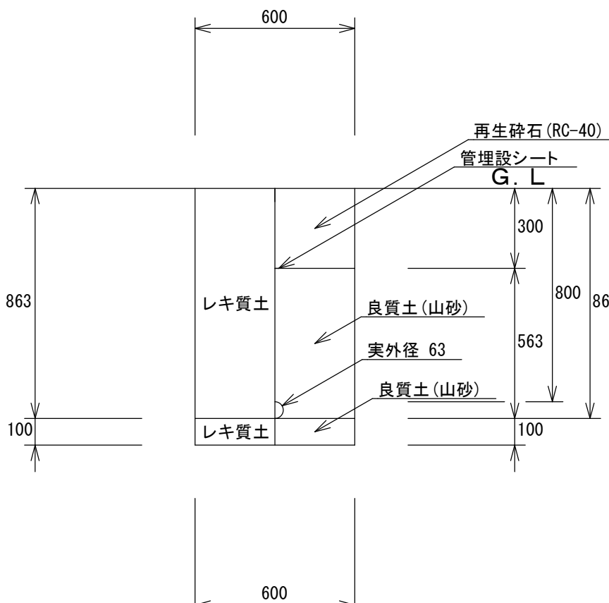
11: 不断水 \phi 125 \times 100 H=0.8m (As) (掘削・埋戻し) 1/20
