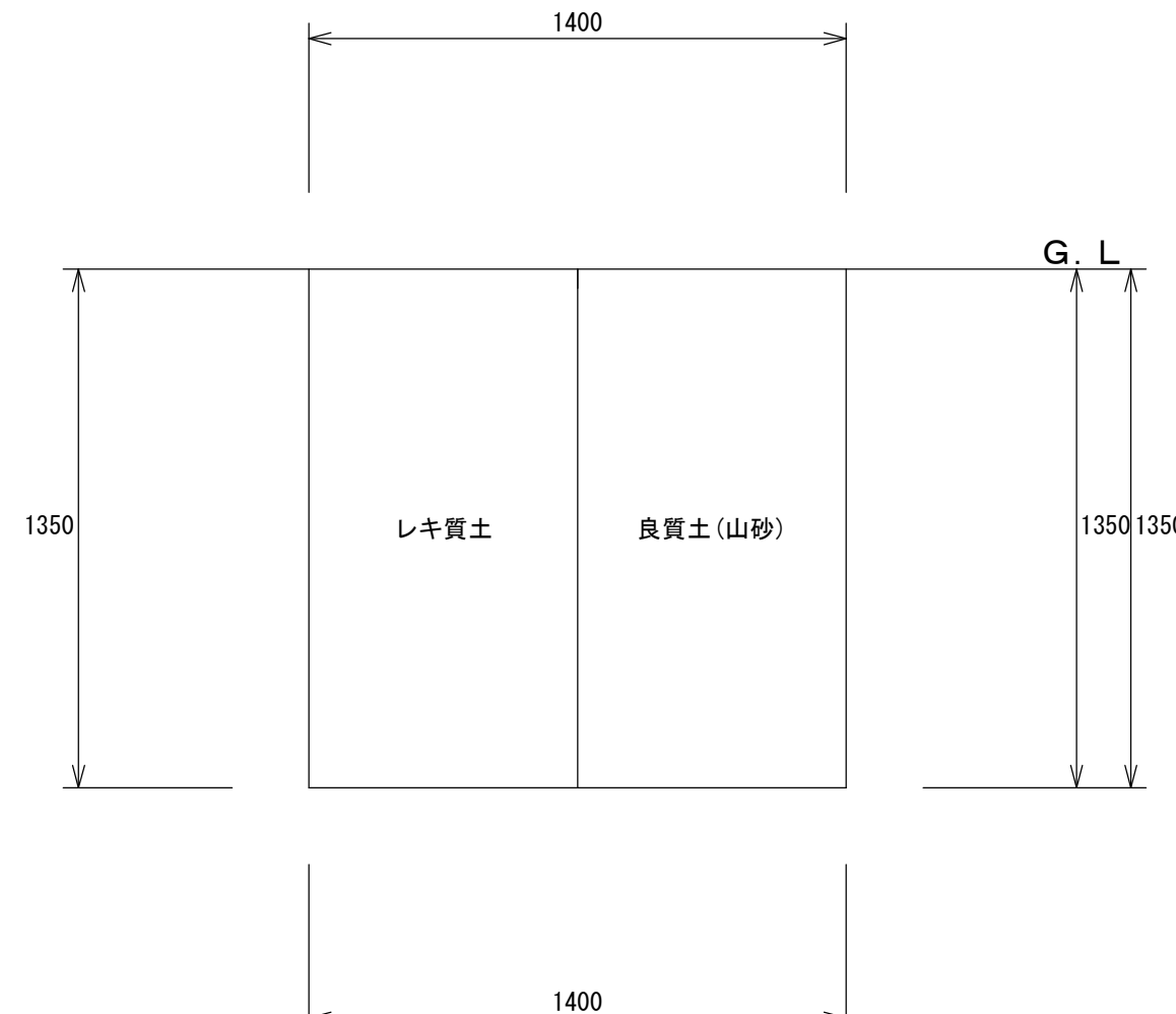
04: PEφ150 H=1.35m (防護コン) (掘削・埋戻し) 1/2
