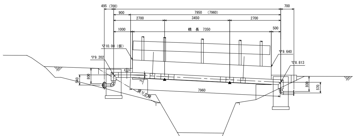
側面図 S= 1:100
