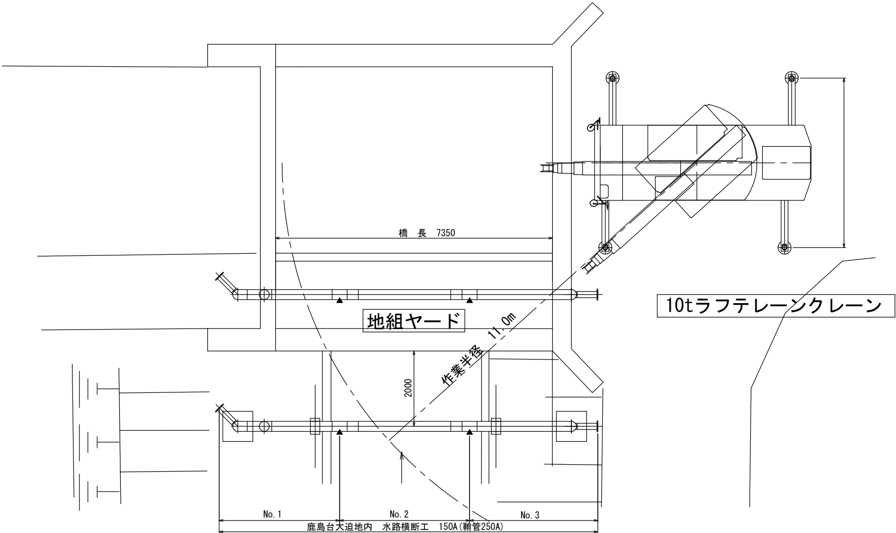
架設計画図 S=1 : 100
