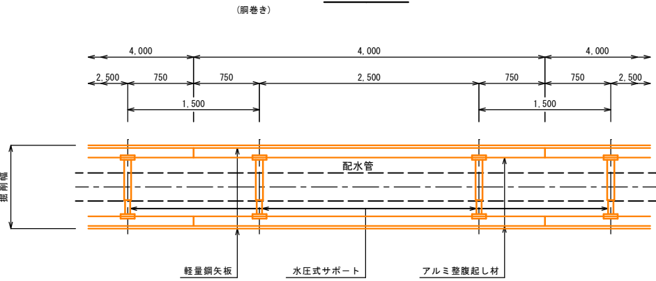
断面図
