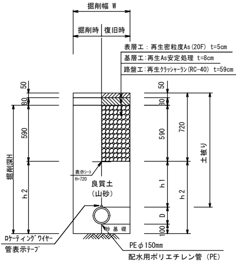
1工区
