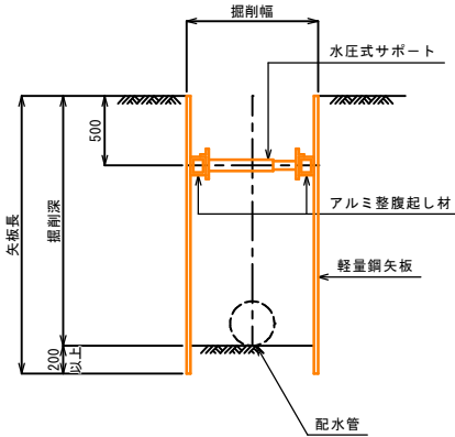
支保工1段
