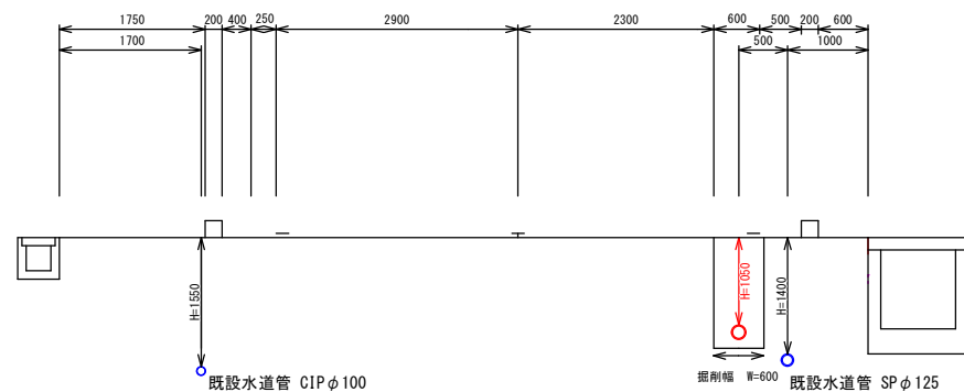
①-①' 断面図
