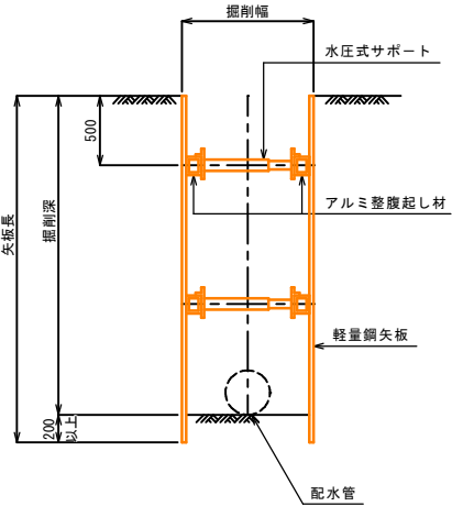
支保工2段
