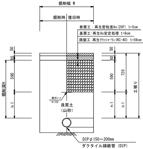
試掘工
