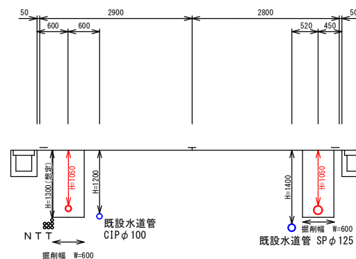
②-②' 断面図
