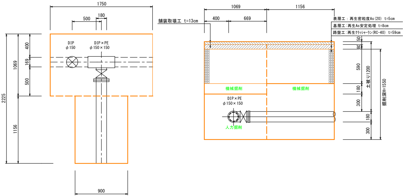
土留工標準図 S=1:30
