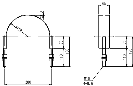
Uバンド詳細図 S=1:5
