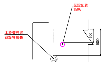
土工部横断図 S=1:30 (A-A)
