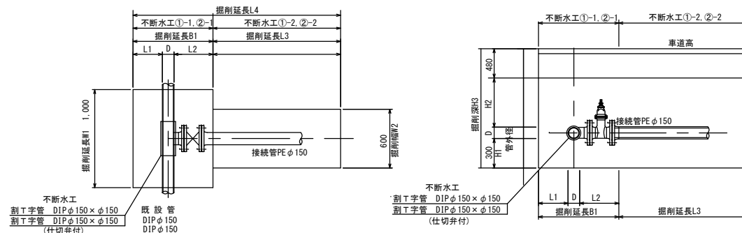
不断水割分岐 寸法表
