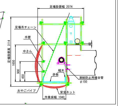
断面図 S=1:30
