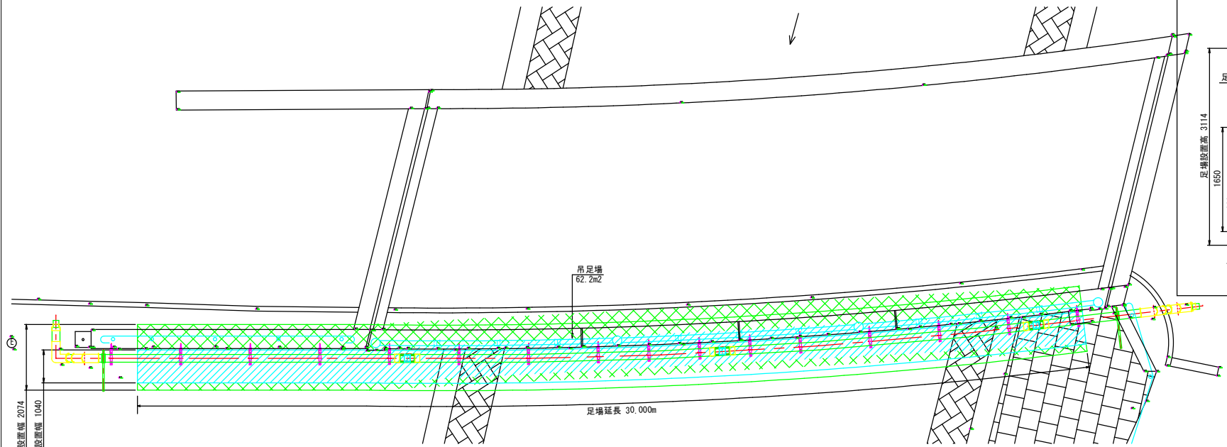
平面図 S=1:60
