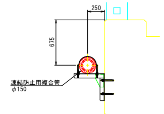
一般断面图 S=1:20
