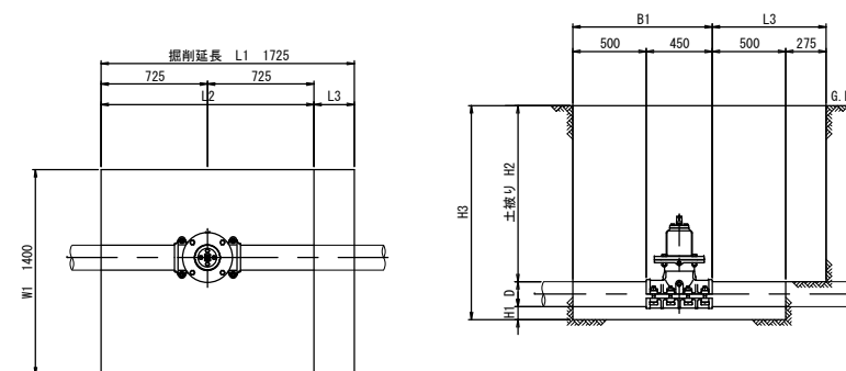
ストッパーバルブ 寸法表
