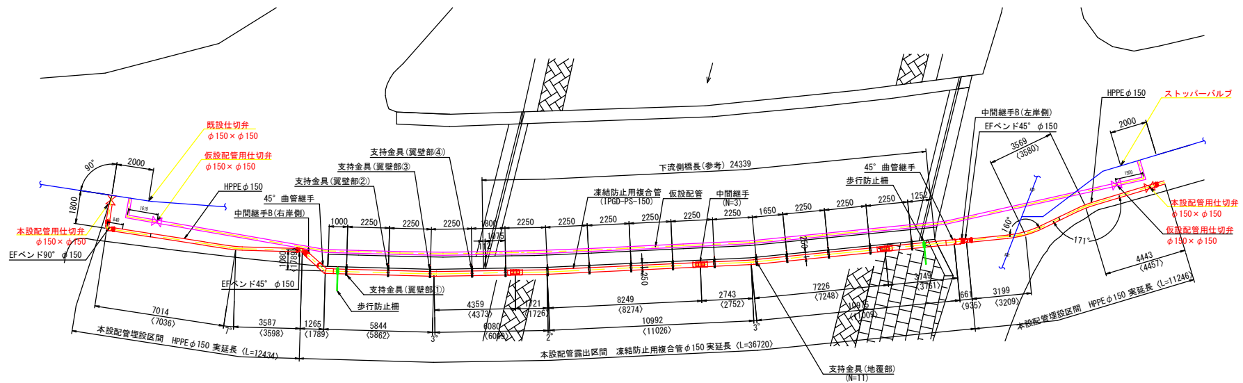
平面図
