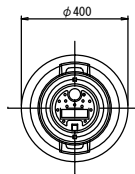
平面図 S=1:10
