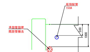
土工部断面図 S=1:30 (A-A)
