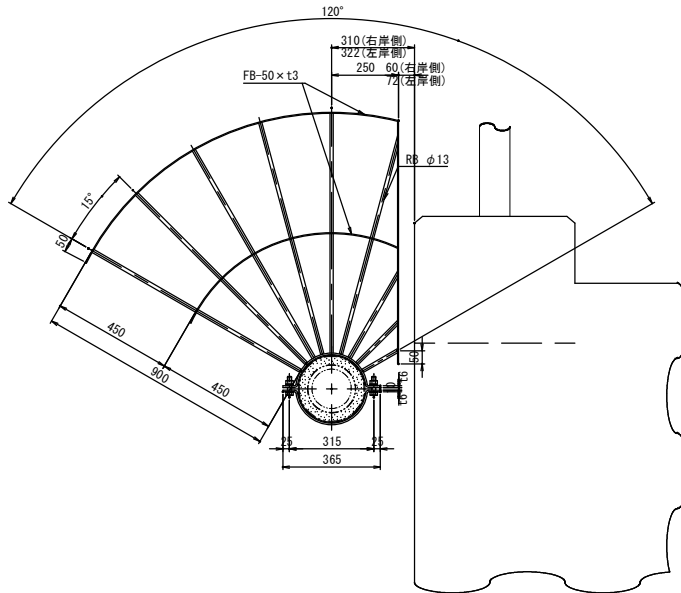
歩行防止柵
