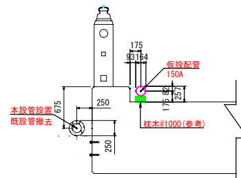
橋面部横断図 S=1:30 (C-C)
