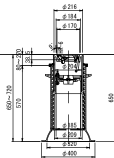
断面図 S=1:10
