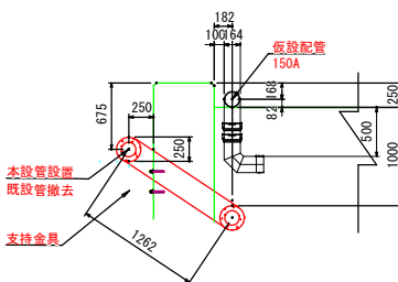
土工部断面図 S=1:30 (B-B)
