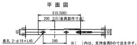
支持金具A(B) SUS304
