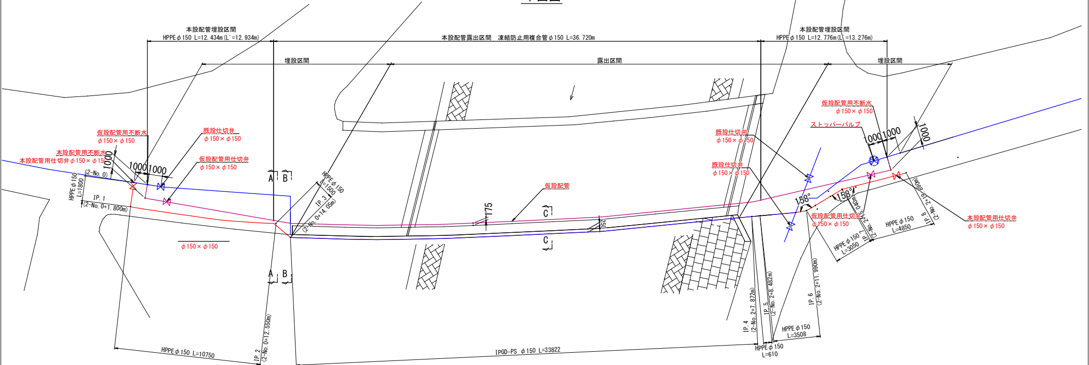
平面図
