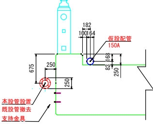
橋面部断面図 S=1:30 (C-C)
