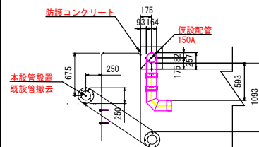
土工部横断図 S=1:30 (B-B)
