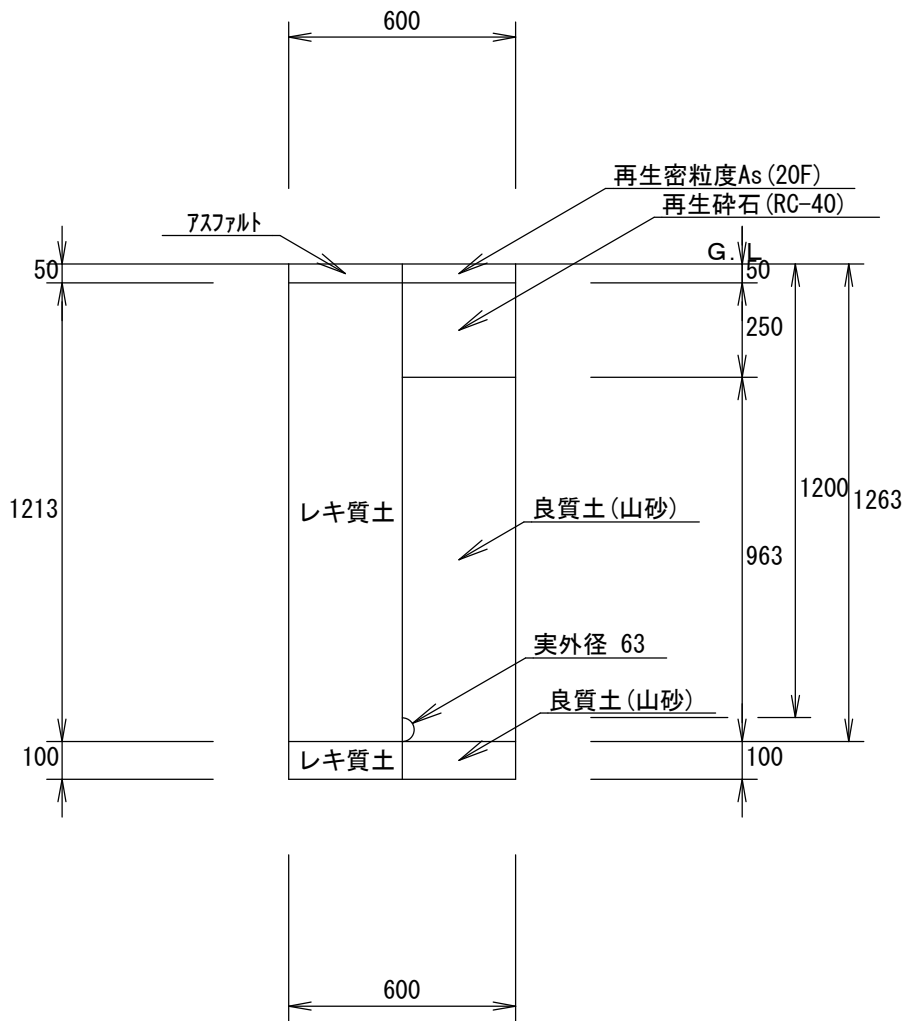
配水管 ③PEφ50 H=1.2m (掘削・埋戻し) 1/20
