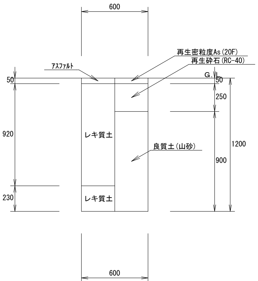
配水管 ⑦試験 H=1.2m (掘削・埋戻し) 1/20
