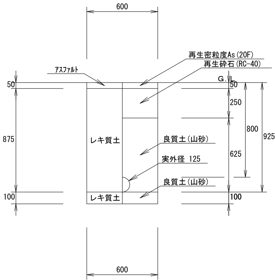
配水管 ②PEφ100 H=0.8m (掘削・埋戻し) 1/20
