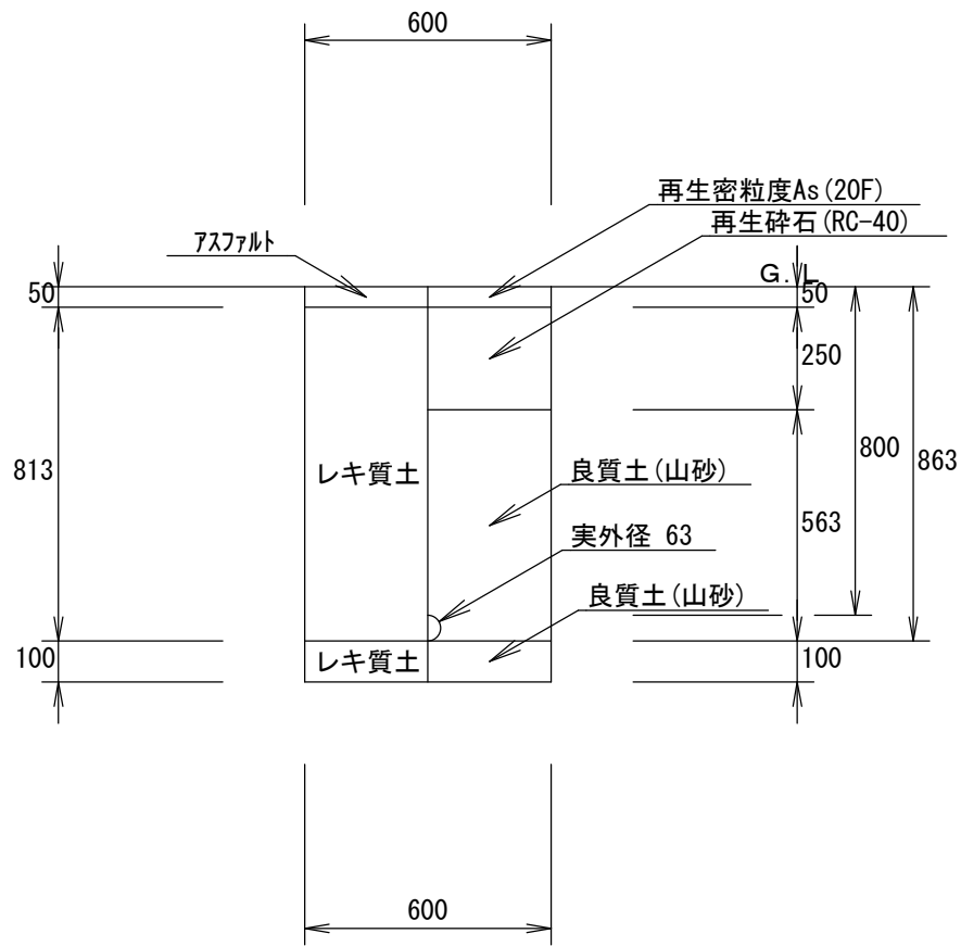
配水管 ④PEφ50 H=0.8m (掘削・埋戻し) 1/20
