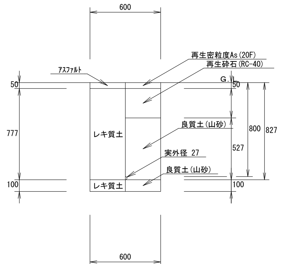
分水管 ①PPφ20 H=0.8m (掘削・埋戻し) 1/20
