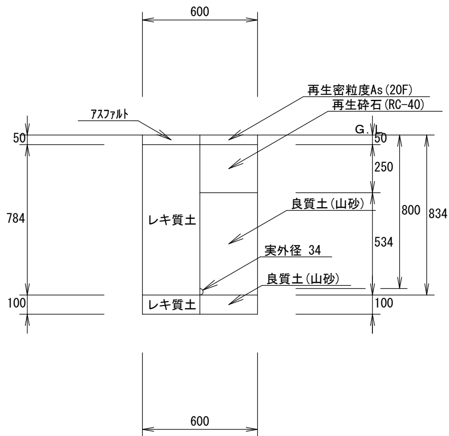
分水管 ②PPφ25 H=0.8m (掘削・埋戻し) 1/20
