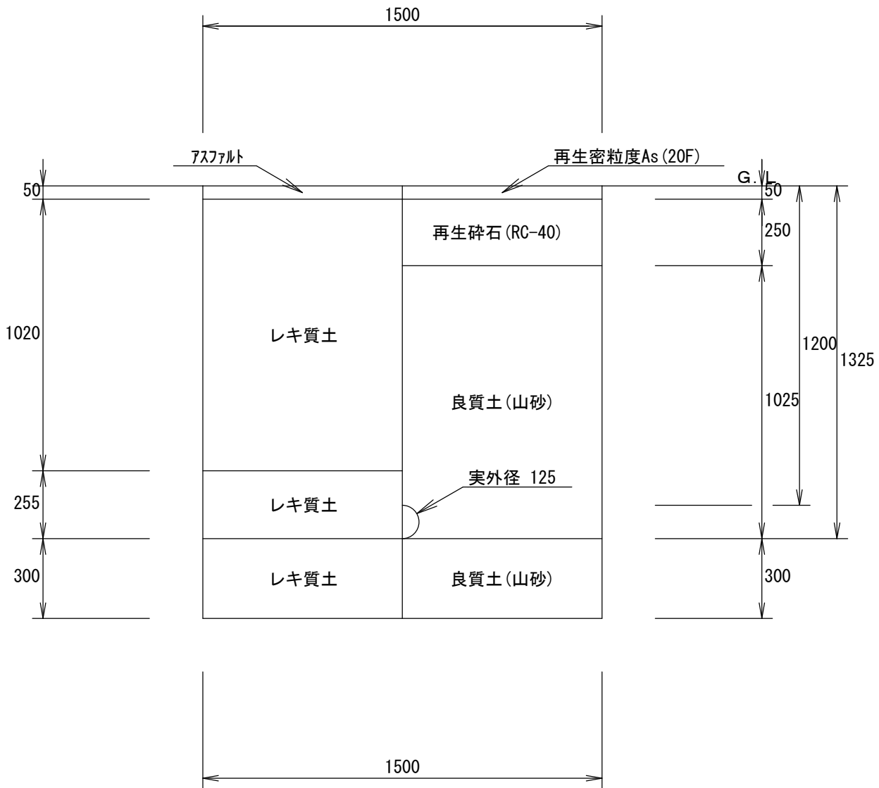
配水管 ⑤不排水 H=1.2m (掘削・埋戻し) 1/20 (掘削深 1.5m以上 土留工あり)
