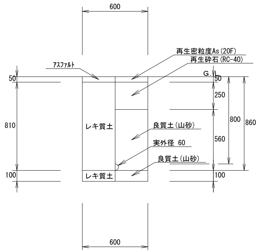
配水管 ⑥VPφ50 H=0.8m (掘削・埋戻し) 1/20
