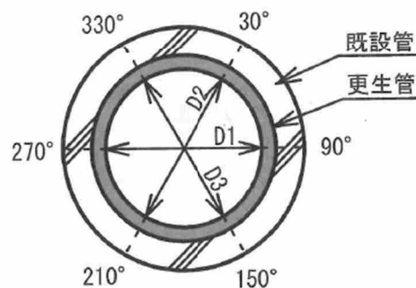
(図 管きょ測定箇所図)
