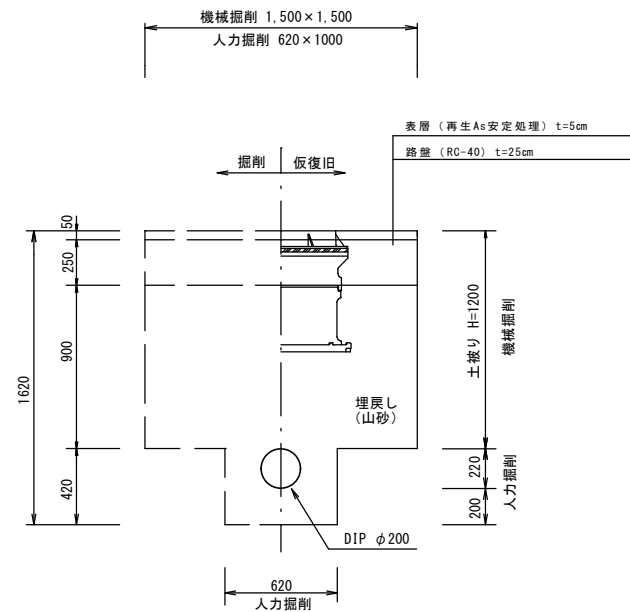
土工標準断面図 S=1/20
