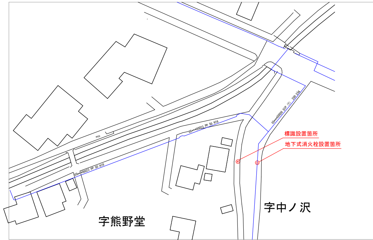
平面図 S=1/500
