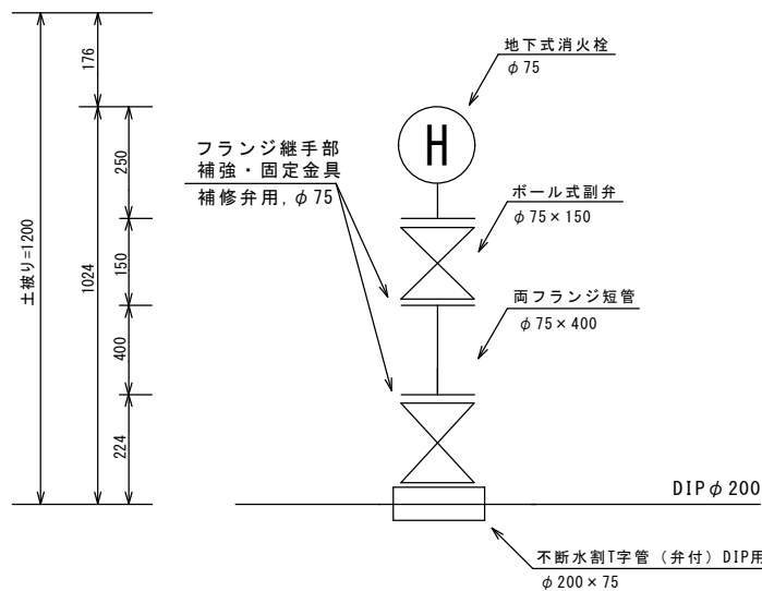
消火栓詳細図 S=free
