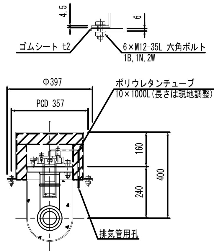
カバー A 詳細 S=1:5
