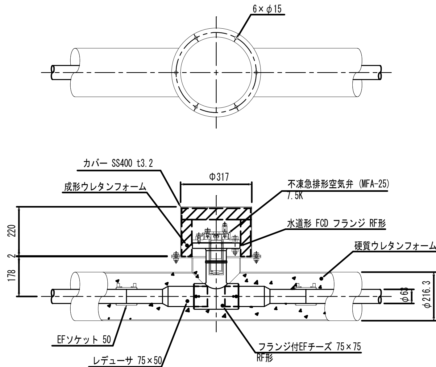
空気弁部詳細図 S=1:10 数量 : 1箇所
